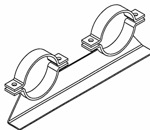
Abstützung „Schelle-Schelle“ Tube support bracket
