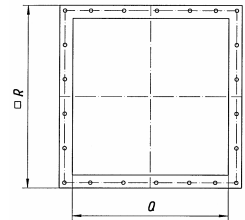
Auslaufflansch Outlet flange
